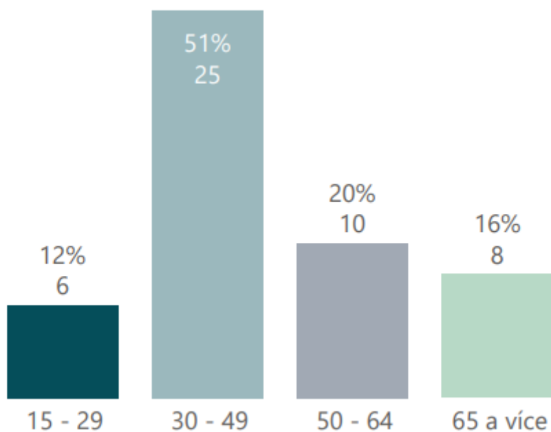
Graf 5: Otázka - Jaký je Váš věk?
